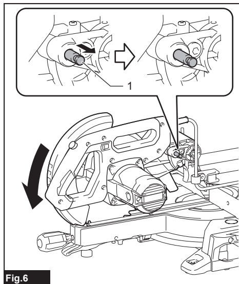
► 1. Clavija de retención
