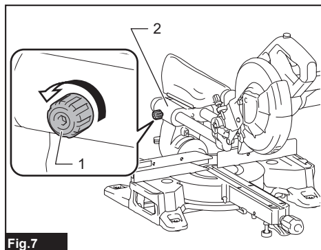
► 1. Tornillo de mariposa 2. Brazo de la herramienta
